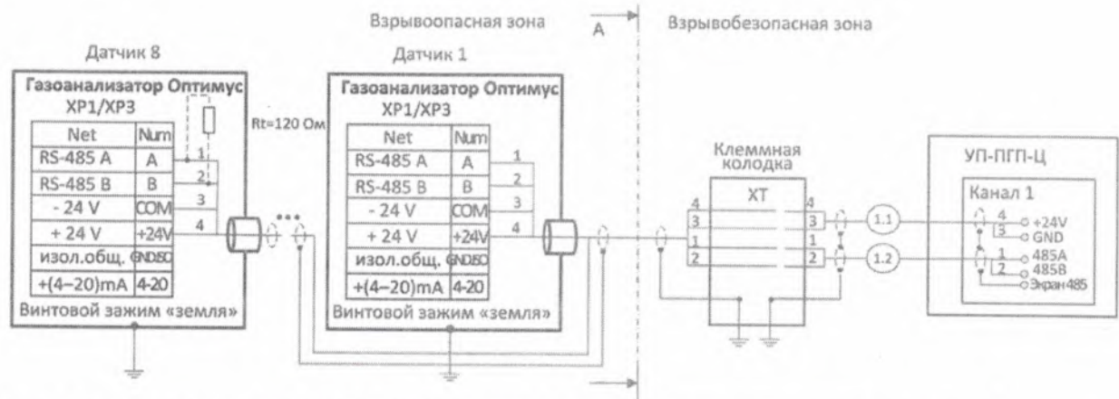
Рисунок А.7 – Схема электрическая трёхпроводная подключения газоанализатора с использованием неизолированной токовой петли к УП-ПГП-А.
