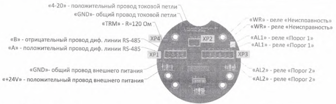
Рисунок 11 – Схема электрическая монтажная (клеммная плата вариант 2 1 )
