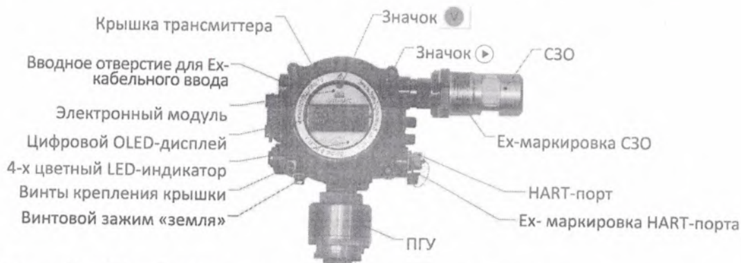
Рисунок 2 – Общий вид газоанализаторов в корпусе с 5-ю вводными отверстиями и дополнительными принадлежностями
