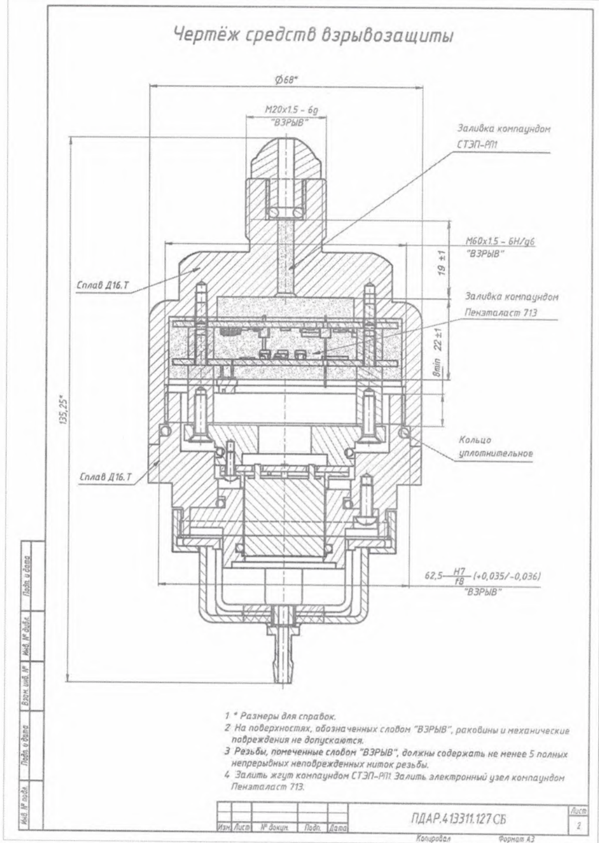
Рисунок Б.3 – Чертеж средств взрывозащиты ППУ
