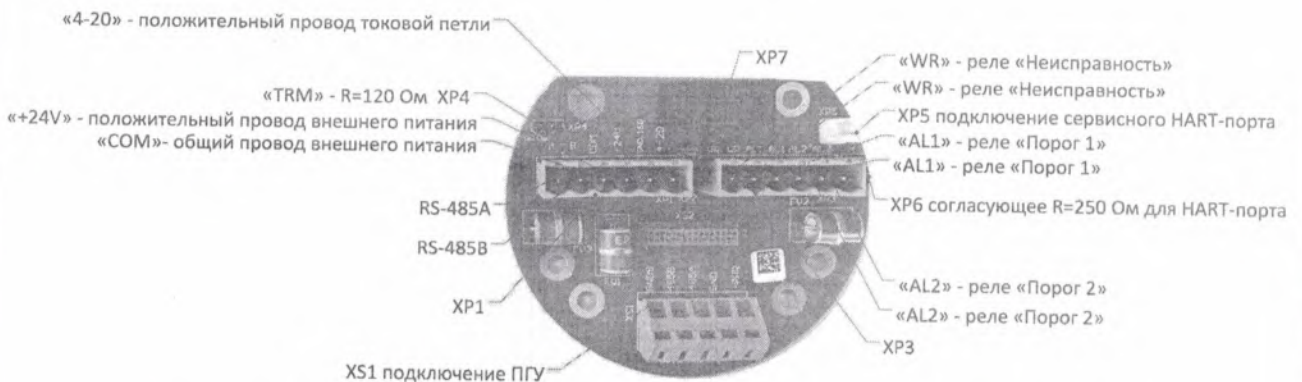
Рисунок 13 – Схема электрическая монтажная (клеммная плата вариант 2 3 )
