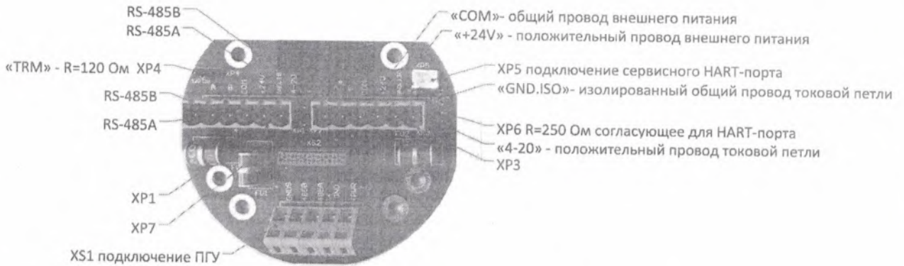
Рисунок 11 – Схема электрическая монтажная (клеммная плата вариант 2 1 )
