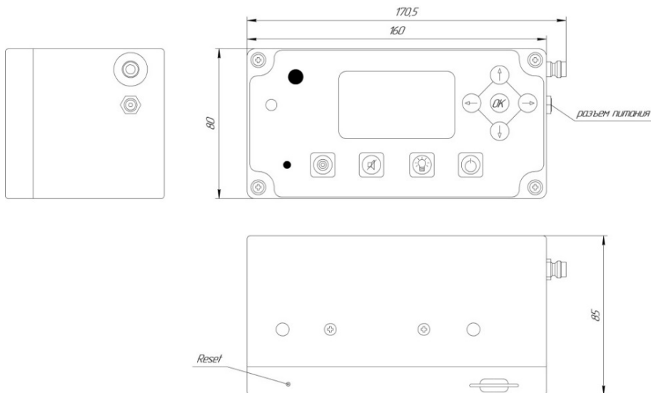
Рисунок 1. Габаритный чертёж прибора
