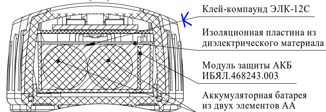
А-А (2:1)
