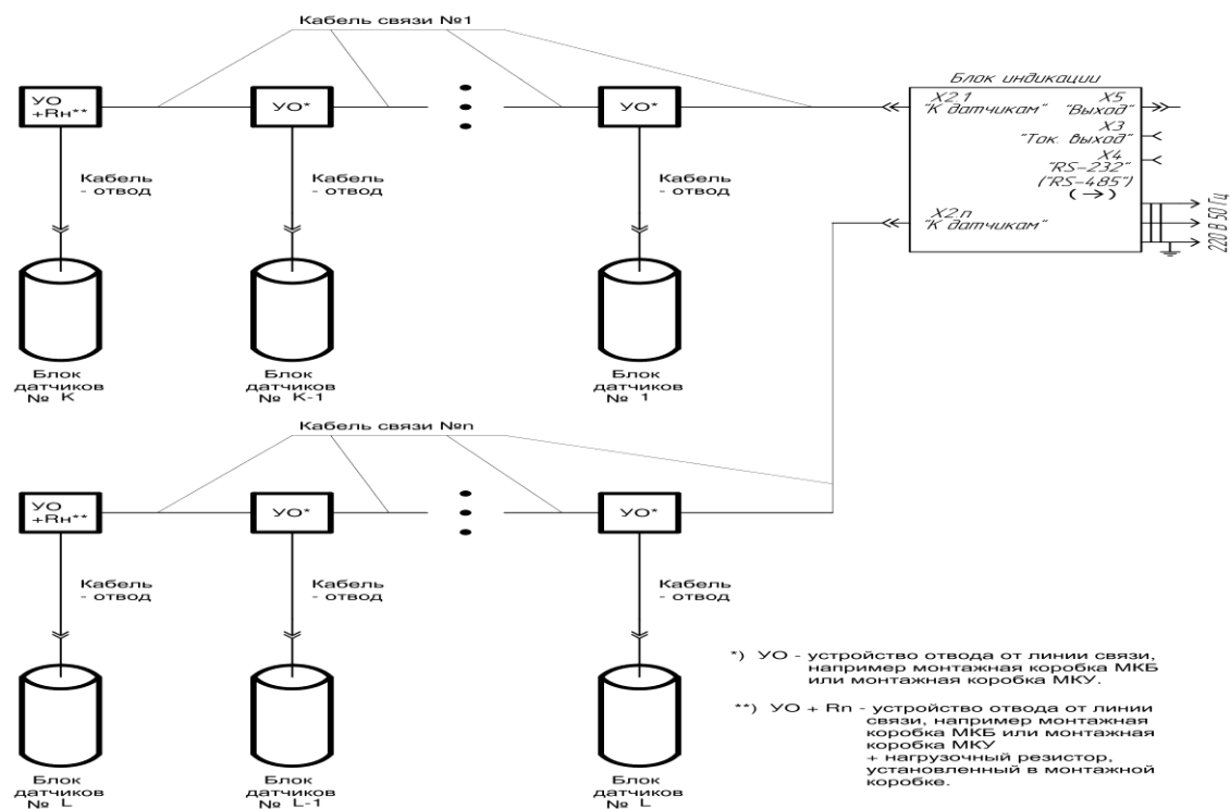
Рис Д.1 Схема соединения "Гирлянда".
