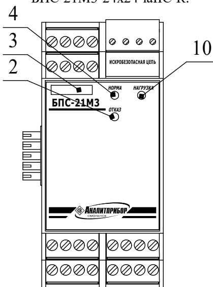
БПС-21М3-24х16-ibПС-К, БПС-21М3-24х24-iaПС-К.
