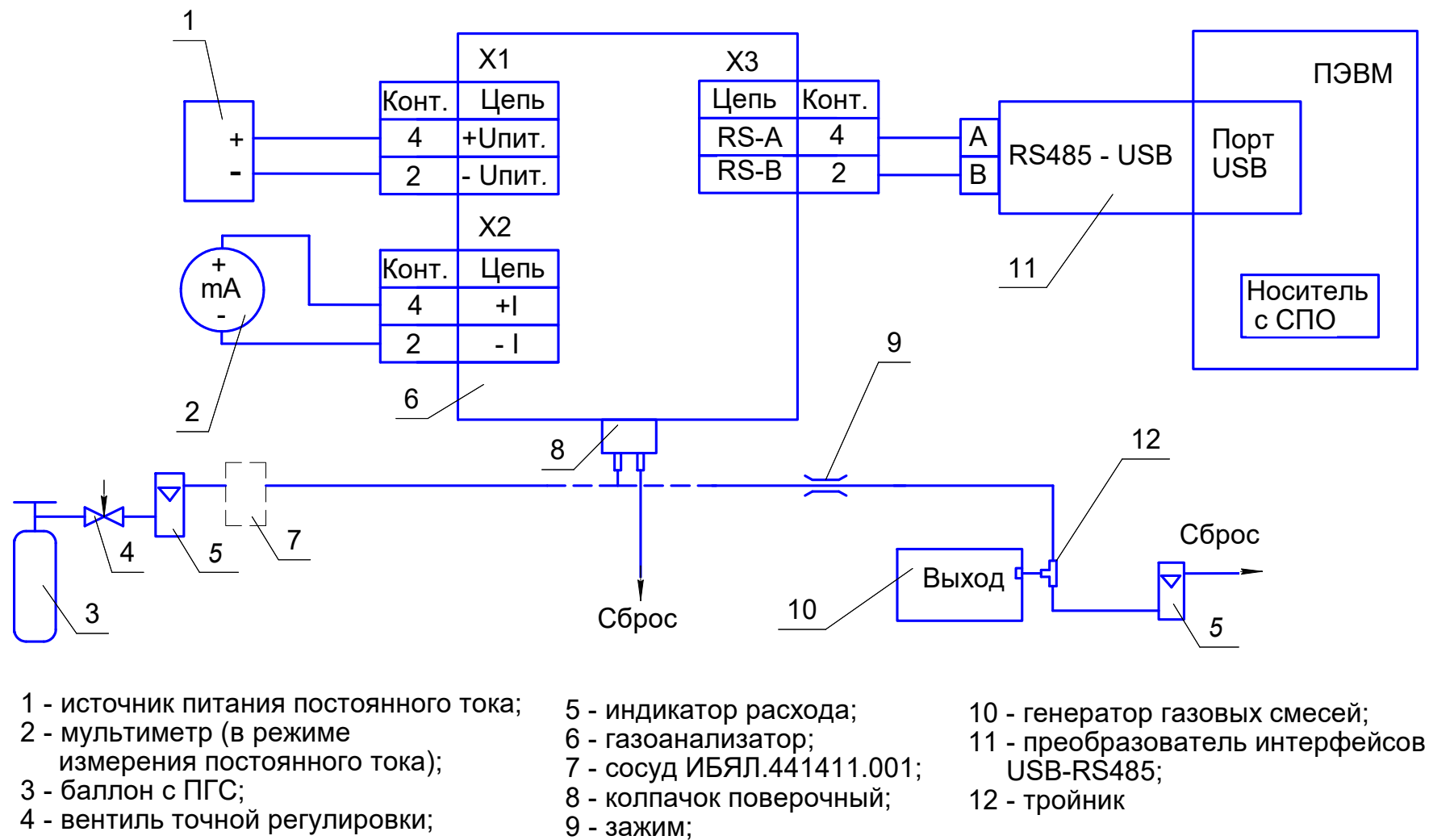
Рисунок К.4 – Схема проверки по ПГС газоанализаторов ДАХ-M-06ТР
